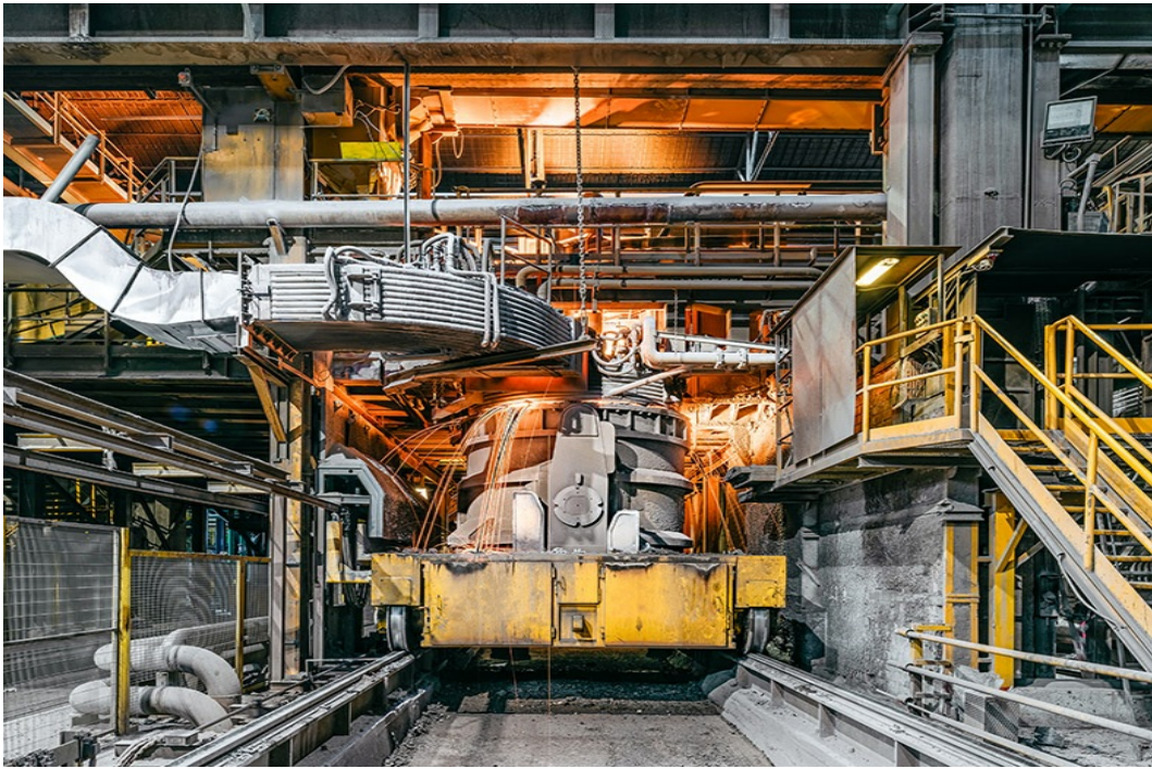
Copyright © Alessandro Roncaglione, Ori Martin, forno di affinazione LF2 per la messa a punto metallurgica degli acciai.
